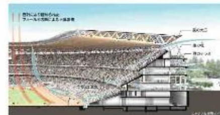
スタジアム断面イメージ
